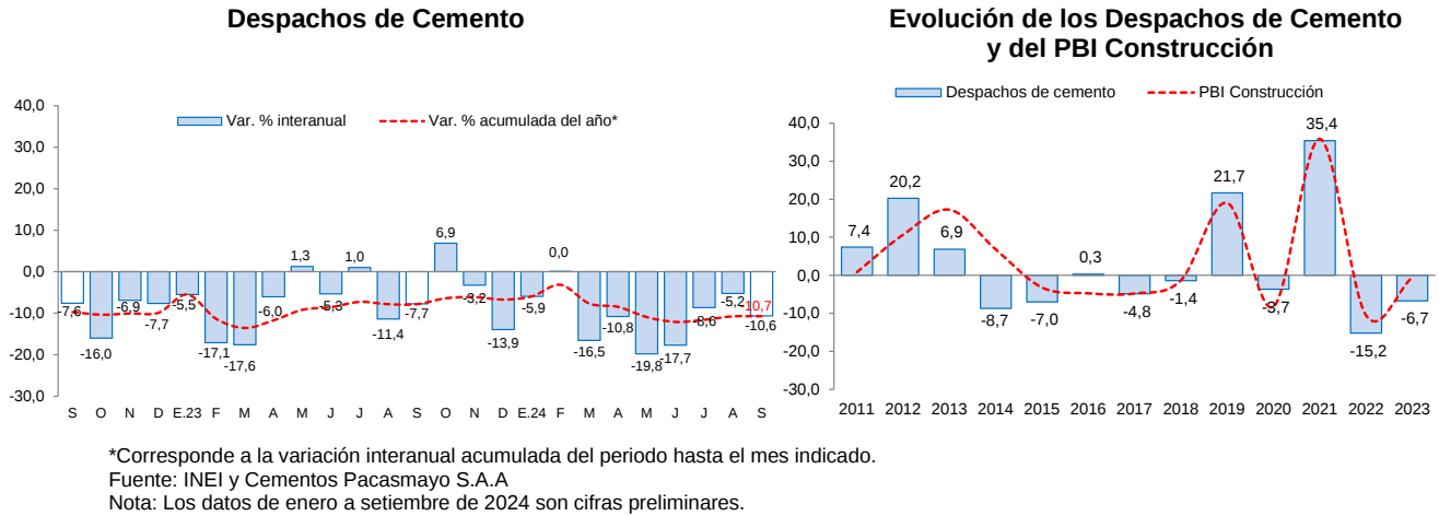
GRÁFICO N° 08 LA LIBERTAD: SECTOR CONSTRUCCIÓN (Variación % real respecto a similar periodo del año anterior)
