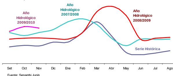
GRÁFICO N° 5 NIVEL DEL AGUA DE RÍO MANTARO
