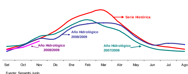
GRÁFICO N° 6 NIVEL DEL AGUA DEL RÍO PERENÉ
