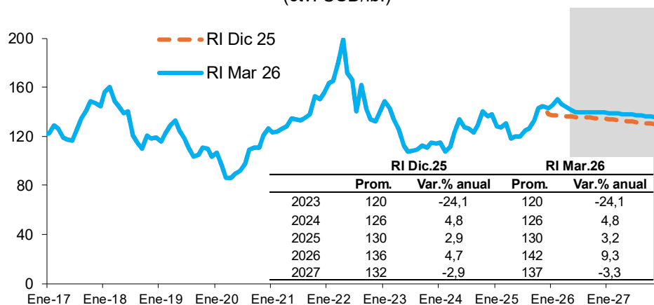
Gráfico 34 ZINC: ENERO 2017 - DICIEMBRE 2027 (ctv. USD/lb.)
