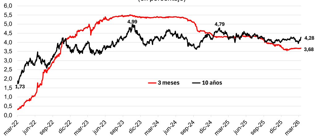
Gráfico 26 Rendimientos de los bonos soberanos de EUA (en porcentaje)
