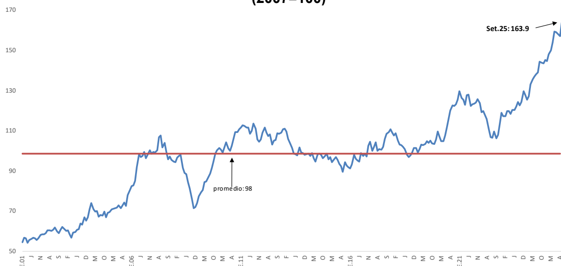
Gráfico 11 Términos de Intercambio: 2001-2025 (2007=100)
