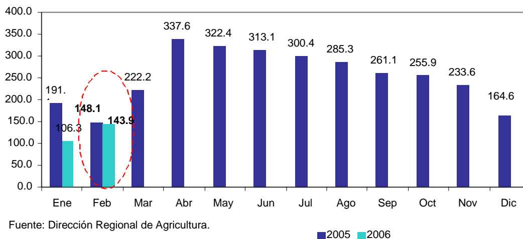
GRÁFICO N° 5 Reservorio Gallito Ciego: Volumen Disponible de Agua (Mill. m3)
