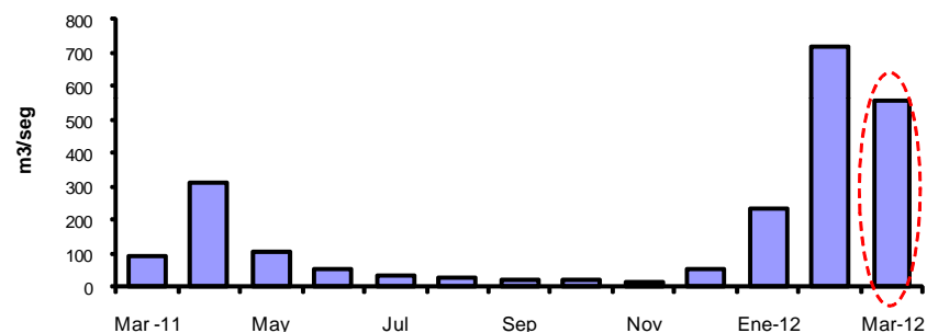
Caudal del río Tumbes
