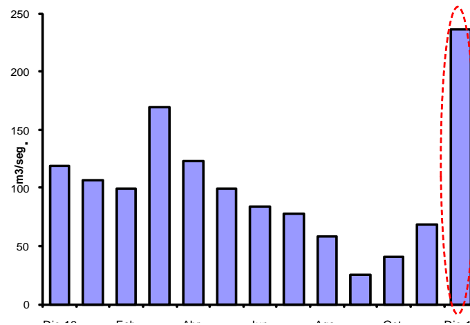
Caudal del río Utcubamba (m 3 /seg.)
