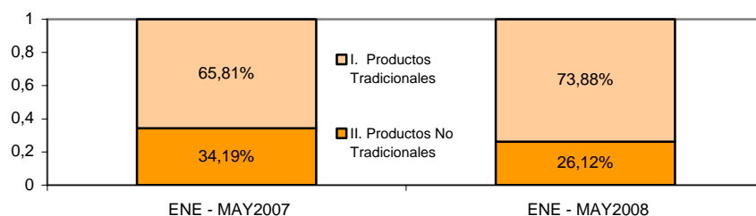
GRAFICO N° 9 ESTRUCTURA DE LAS EXPORTACIONES POR GRUPO DE PRODUCTO
