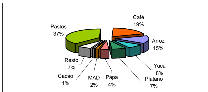
Gráfico Nº 3 PARTICIPACIÓN EN EL VBP AGRÍCOLA (ENERO - MAYO 2008)
