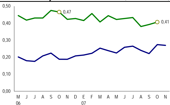
Gráfico N° 8 Diesel 2: Oferta y Demanda en Amazonas (Miles de Barriles x día)
