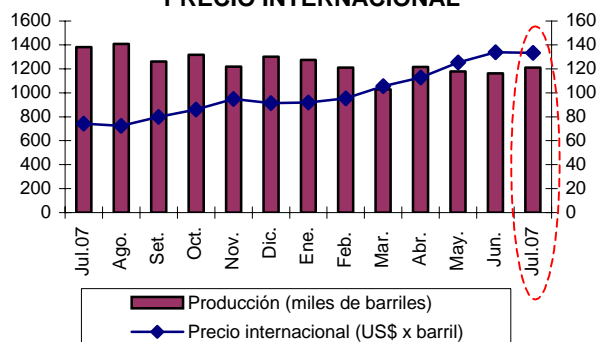
GRÁFICO Nº 5 PRODUCCIÓN DE PETRÓLEO CRUDO Y PRECIO INTERNACIONAL
