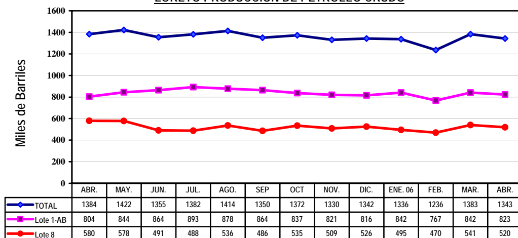
LORETO PRODUCCION DE PETROLEO CRUDO
