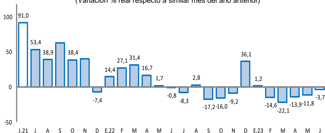
GRÁFICO N° 2 PASCO: CRECIMIENTO DE LOS DESPACHOS DE CEMENTO (Variación % real respecto a similar mes del año anterior)
