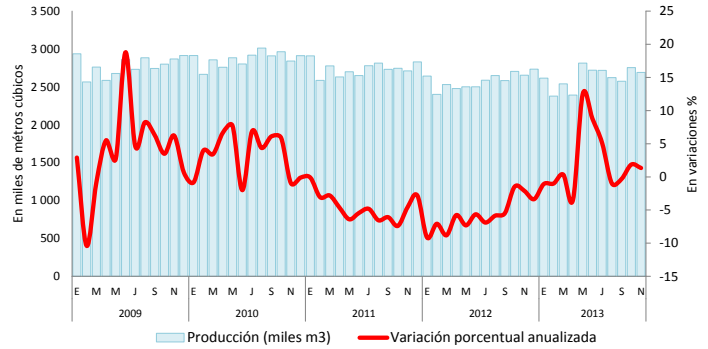
GRÁFICO Nº 26 SEDAM HYO: PRODUCCIÓN DE AGUA POTABLE (Producción en miles de metros cúbicos)
