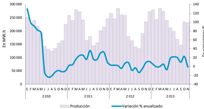
GRÁFICO Nº 25 JUNÍN: PRODUCCIÓN DE ENERGÍA ELÉCTRICA (Producción en MW.h)
