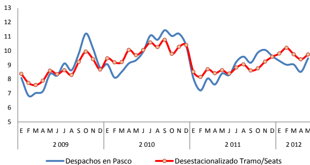
GRÁFICO Nº 13 DESPACHOS DE CEMENTO EN PASCO (En miles de toneladas)
