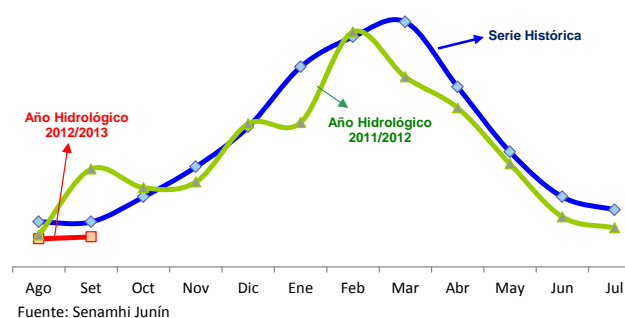
GRÁFICO Nº 15 NIVEL DE AGUA DEL RÍO PERENÉ
