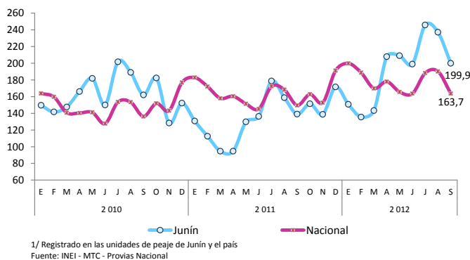
GRÁFICO N° 7 ÍNDICE DEL FLUJO DE VEHÍCULOS LIGEROS 1/ (Año Base 2002 = 100)
