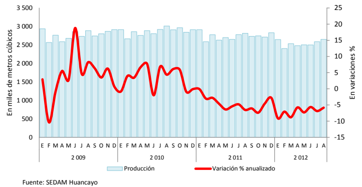
GRÁFICO N° 27 SEDAM HYO: PRODUCCIÓN DE AGUA POTABLE (Producción en miles de metros cúbicos)
