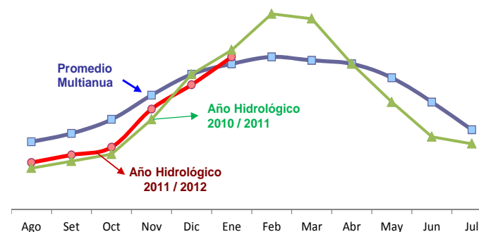
Zona selva: Nivel del río Huallaga en la estación de Tingo María
