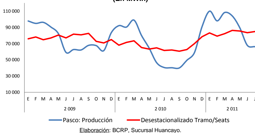
GRÁFICO N° 16 PRODUCCIÓN DE ENERGÍA ELÉCTRICA (En MW.h)
