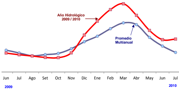
GRÁFICO N° 11 NIVEL DEL AGUA DE RÍO HUALLAGA ZONA SIERRA – ESTACIÓN SAN RAFAEL
