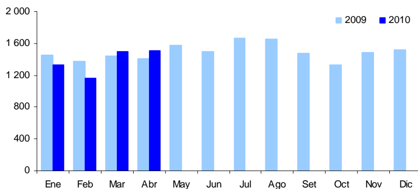
GRÁFICO N° 6 GENERACIÓN ELÉCTRICA (Megavatios Hora)
