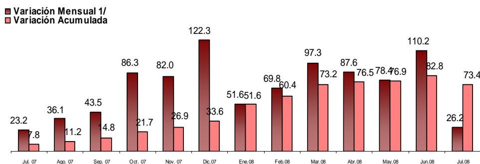
GRÁFICO N° 8 VALOR BRUTO DE LA PRODUCCIÓN MINERA 2007 – 2008
