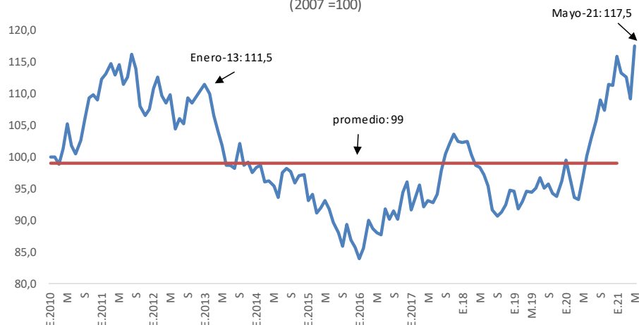
Gráfico 15 Términos de Intercambio 2010-2021 (2007 =100)
